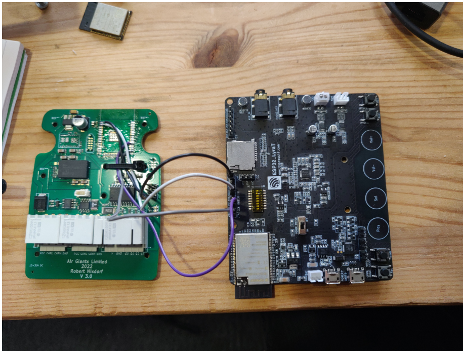
MTDI (GPIO_12) → CAN_D
